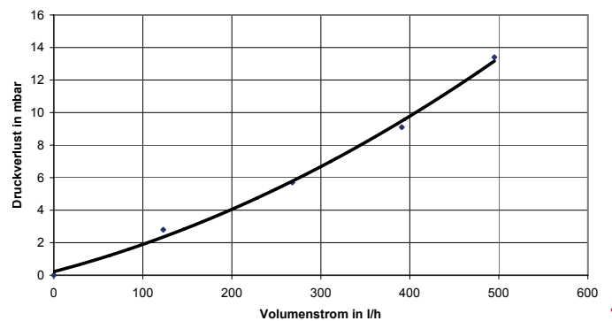
Druckverlust RA 251-4
