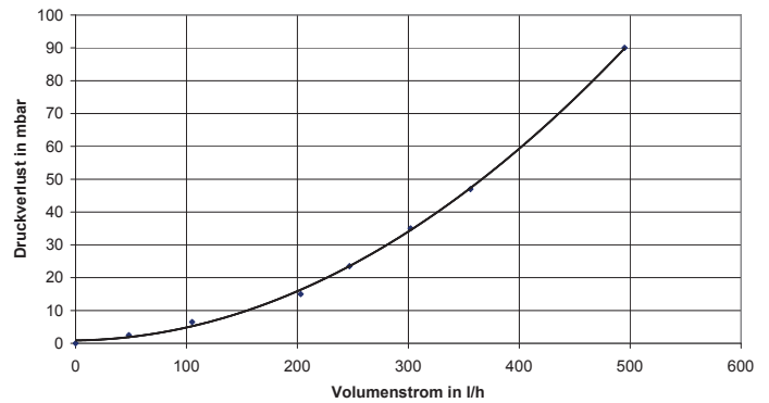
Druckverlust RA 215
